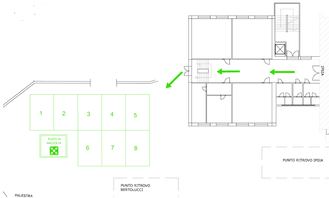
Figura 3: pianta piano rialzato
