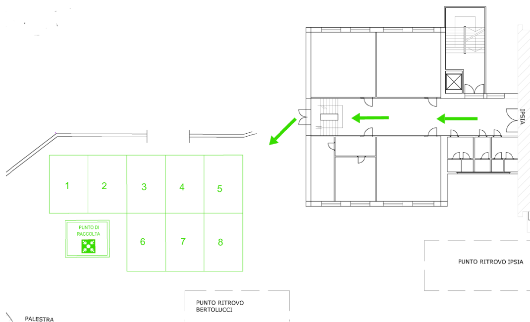
Figura 3: pianta piano rialzato
